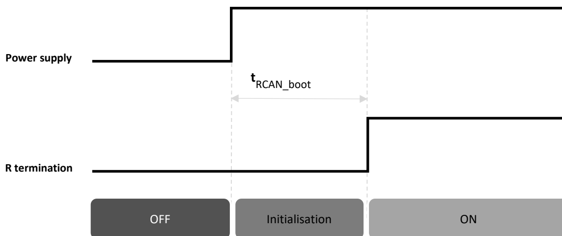
Figure 16 - Diagramme d'initialisation du bus CAN
