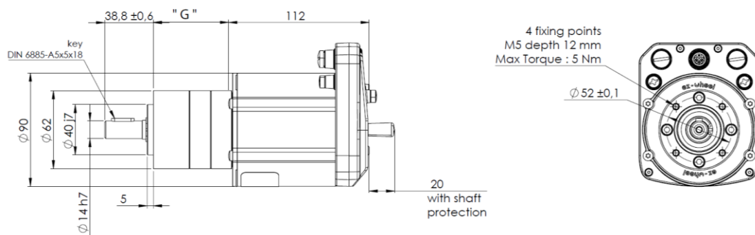
Figure 9 - Dimensions hors tout – SWD® Core avec réducteur(s)
