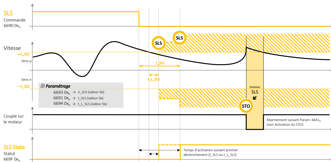
Figure 38 - Diagramme d'activation du SLS
