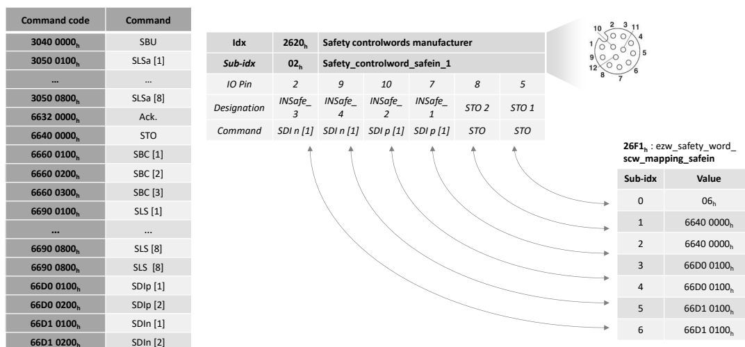
Figure 35 - Exemple de configuration des commandes de sécurité par les SafeInputs
