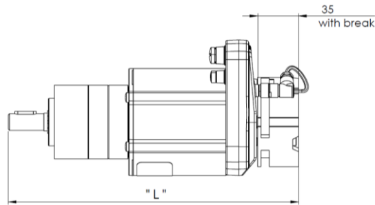
Figure 10 - Dimensions hors tout - SWD® Core - avec frein externe
