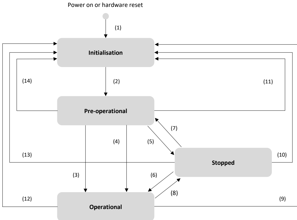
Figure 17 - Diagramme de machine à état NMT d'un périphérique CANopen
