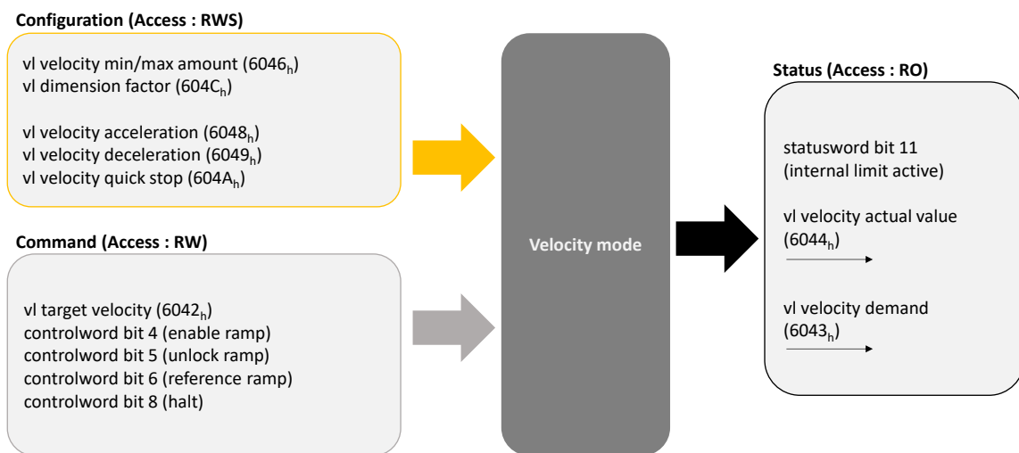
Figure 26 - Interface du 'contrôle en vitesse'
