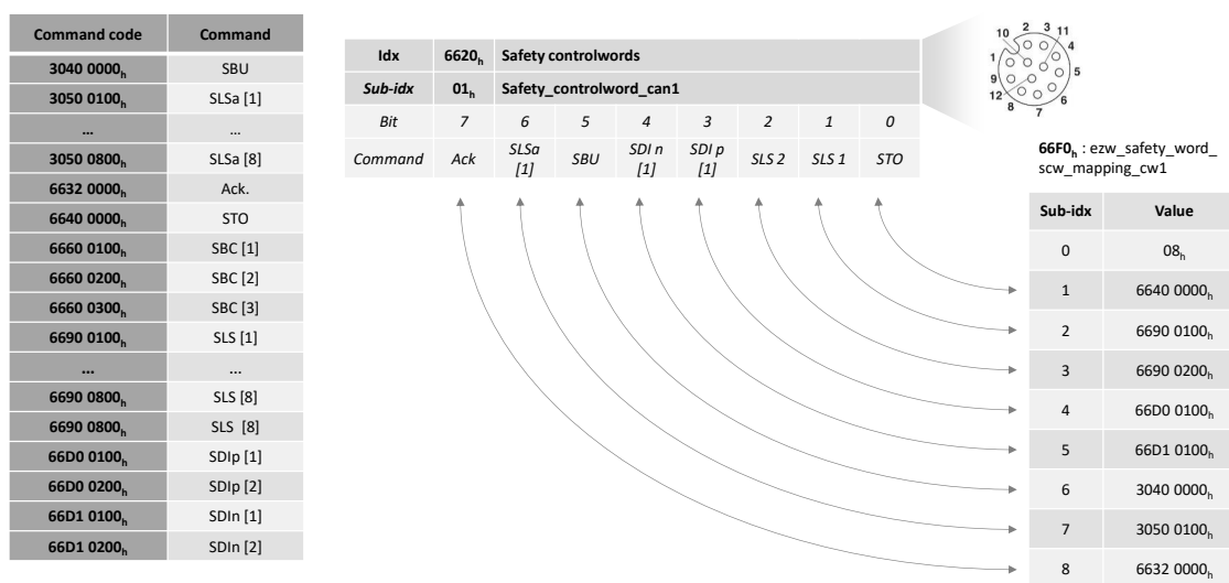
Figure 34 - Exemple de configuration des commandes de sécurité par le CANopen
