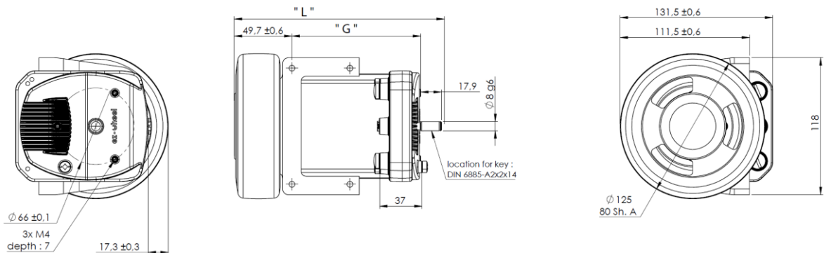
Figure 11 - Dimensions hors tout – 'SWD® 125 1-stage'
