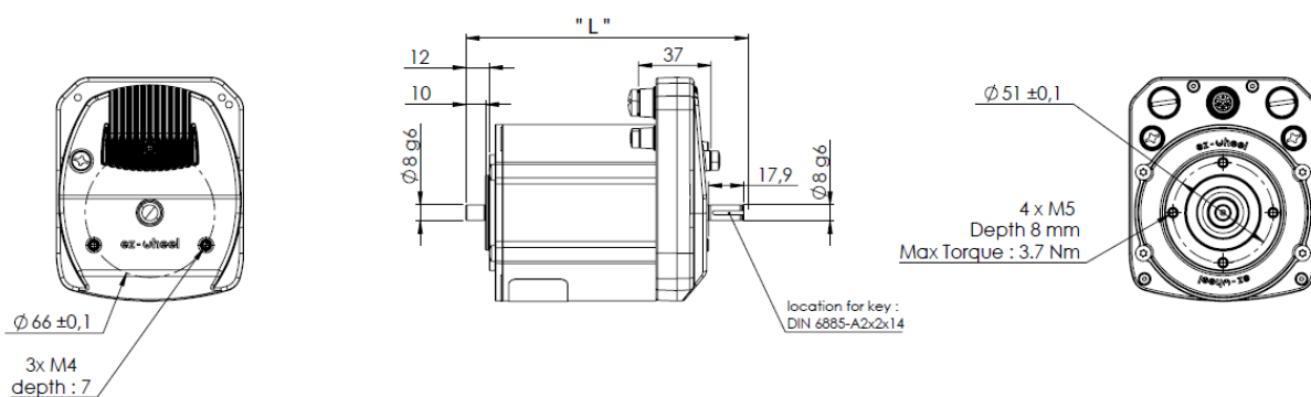
Figure 8 - Dimensions hors tout – SWD® Core nu
