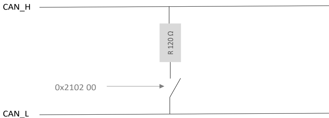
Figure 15 - Activation de la résistance de terminaison interne
