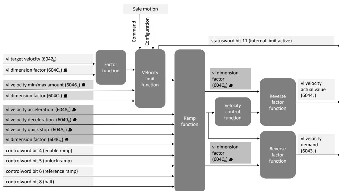
Figure 27 - Architecture 'contrôle en vitesse'
