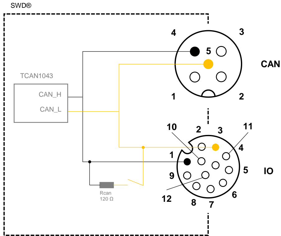
Figure 14 - Schéma électrique interne du bus CAN
